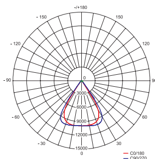
Тип Г (60°)
