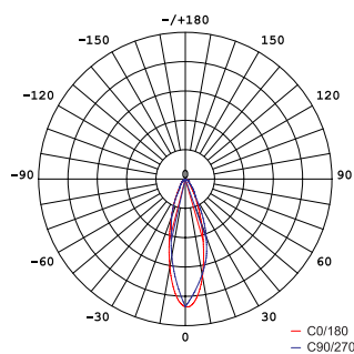
Тип К (30°)
