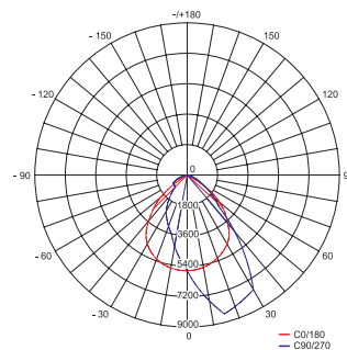
Тип «Кососвет»
