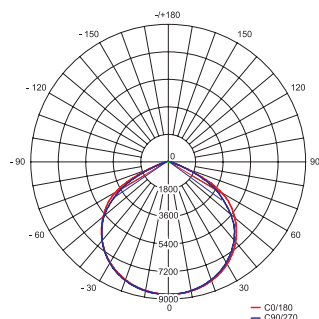
Тип Д (120°)
