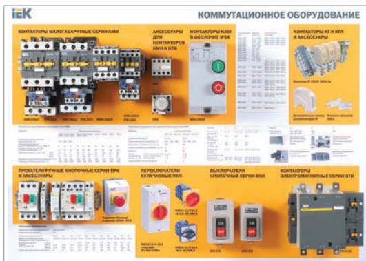
Коммутационное оборудование
