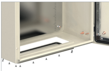
Съемные кабельные фланцы удобный ввод кабеля (для корпусов глубины от 200 мм)
