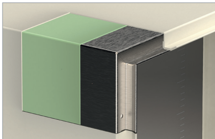
Грунтование перед окрашиванием максимальная защита от коррозии
