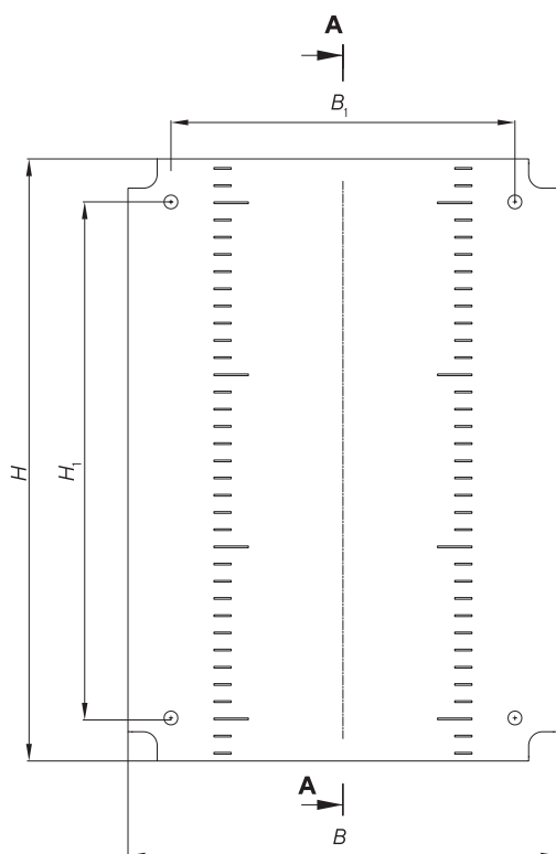
Панель монтажная ЩМП TiTAN
