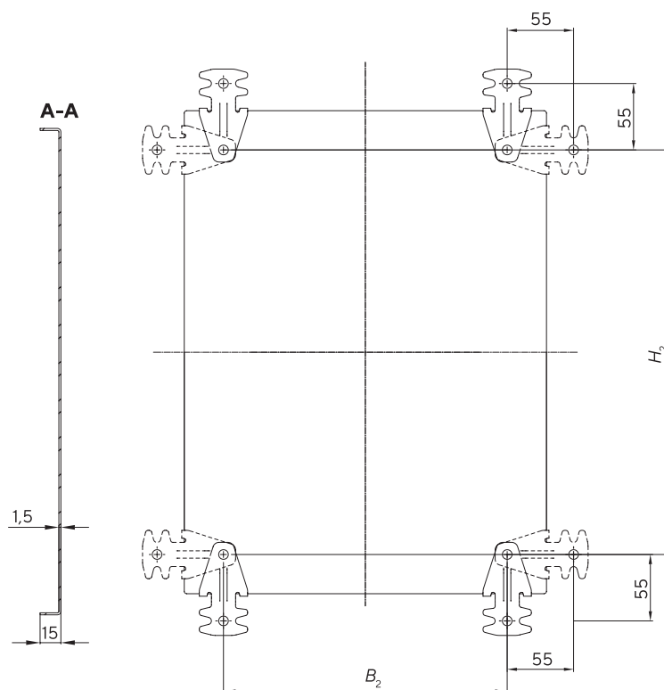
Задняя стенка и комплект для навески
