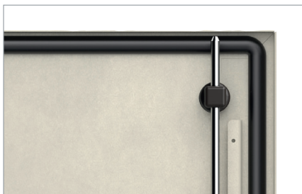
Вертикальные Z-профили на внутренней стороне двери дополнительная жесткость и монтаж оборудования на дверь (для корпусов высотой от 400 мм)
