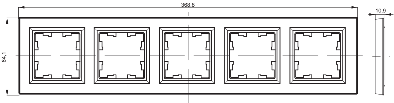
Рамка 5 постов
