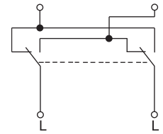
Переключатель одноклавишный
