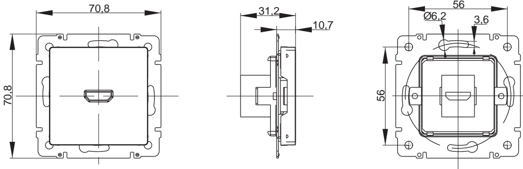
Розетка HDMI
