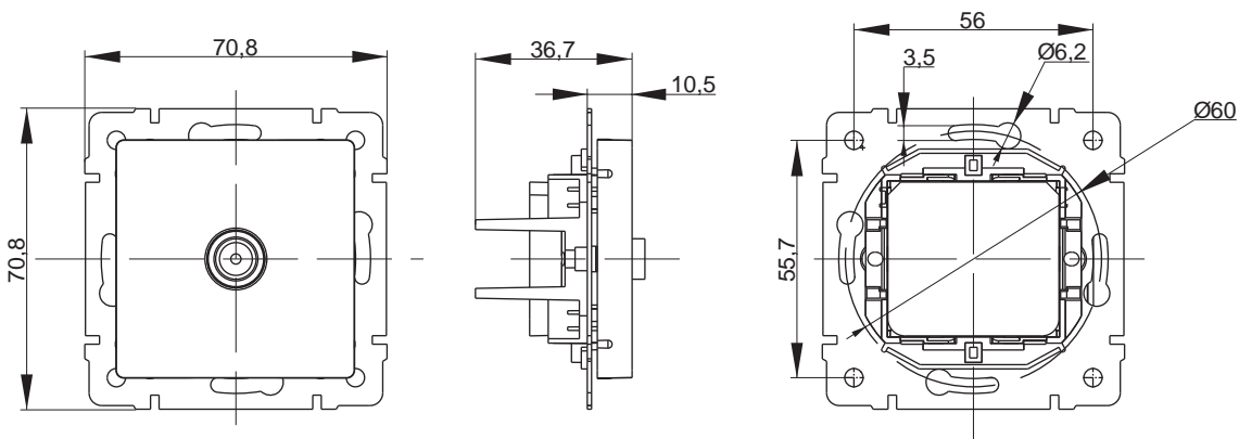
Телевизионная розетка
