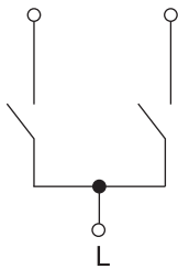
Выключатель двухклавишный
