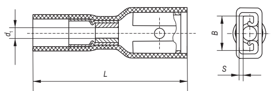
Разъем РпИм-т
