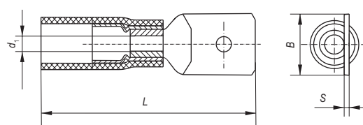
Разъем РпИп-т
