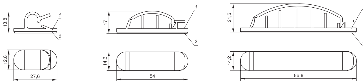
КС-1 1 – изделие; 2 – клейкая лента
