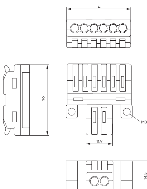
СМК 222-41124, СМК 222-41126
