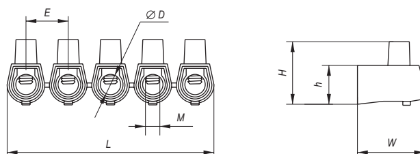
КЗВИ (51)
