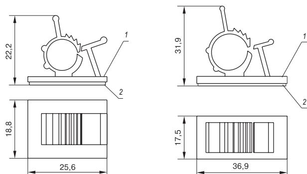
КС-10 1 – изделие; 2 – клейкая лента
