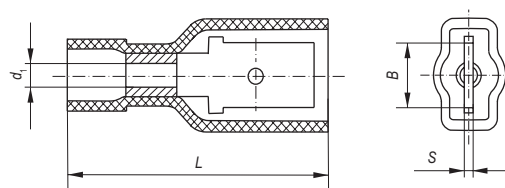
Разъем РпИп-н
