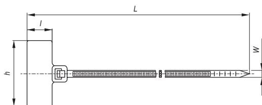
Хомут типа ХП1
