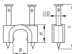
СКК30, СКК35
