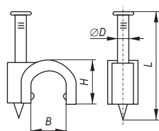
СКК4 ...СКК25
