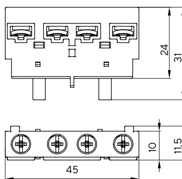
Контакты поперечные
