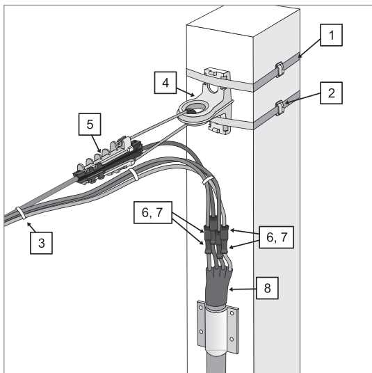
Перечень арматуры, необходимой для монтажа узла на основе провода СИП 3×50+54,6
