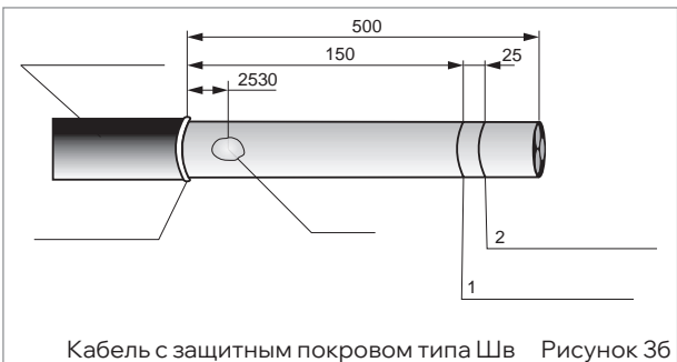
Кабель с защитным покровом типа Шв Рисунок 3б
