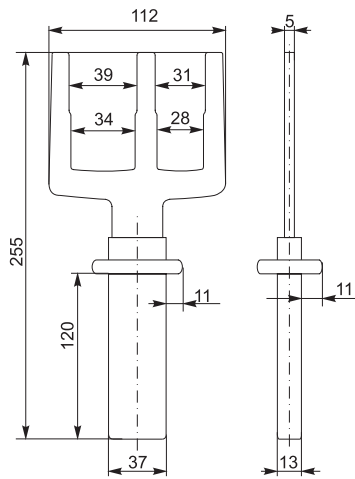
ДЗ-1
