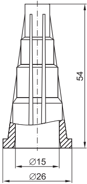
КИ 16 150
