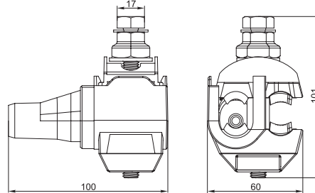
ЗСГП10-120/25-95
