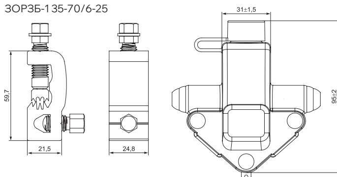
ЗОРЗБ-135-70/6-25
