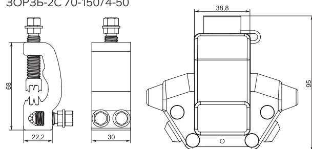
ЗОРЗБ-2С 70-150/4-50
