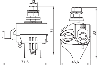
ЗСГП10-95/6-35
