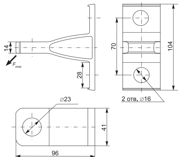
КАМ-1500
