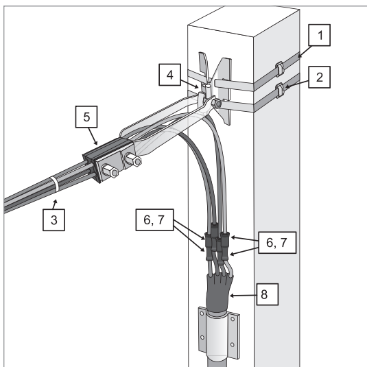
Перечень арматуры, необходимой для монтажа узла на основе провода СИП 4×50
