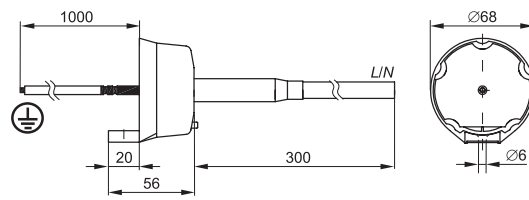
ОПН-XXX Ш
