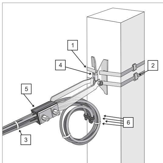
Перечень арматуры, необходимой для монтажа узла на основе провода СИП 4×50+25
