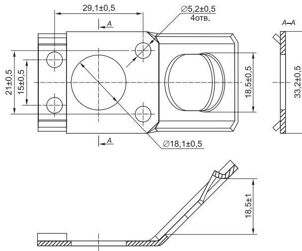
КАБ-200
