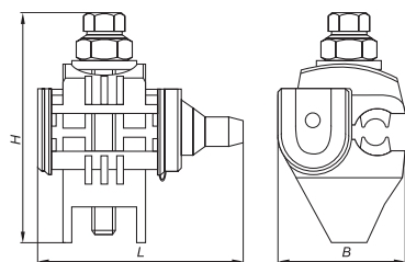
ЗОРЗБ-116-25/4-25
