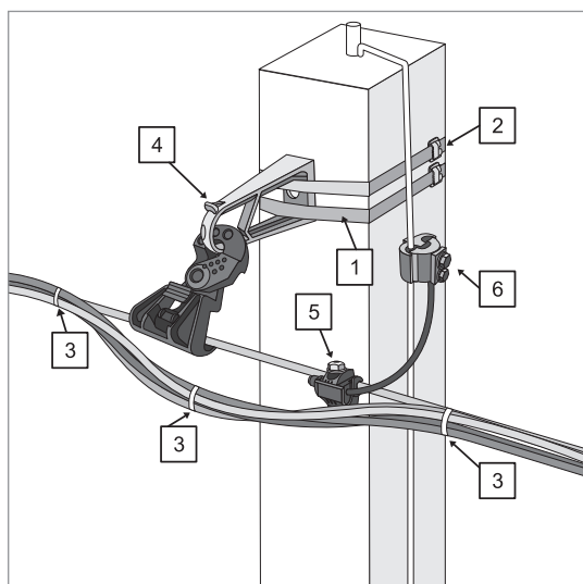
Перечень арматуры, необходимой для монтажа узла на основе провода СИП 3×50+54,6+25
